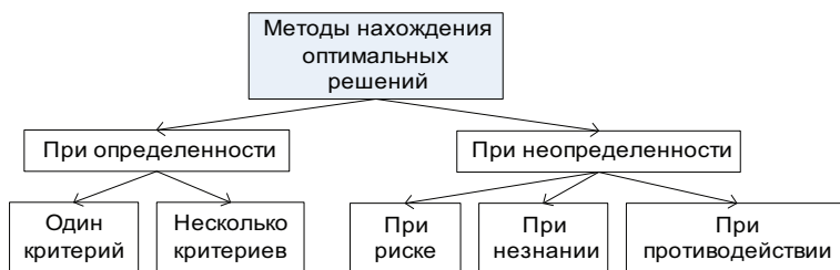
Рис. 1.4. Классификация методов нахождения оптимальных решений
