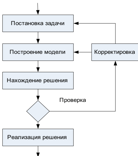
Рис. 1.2. Алгоритм операционного исследования
