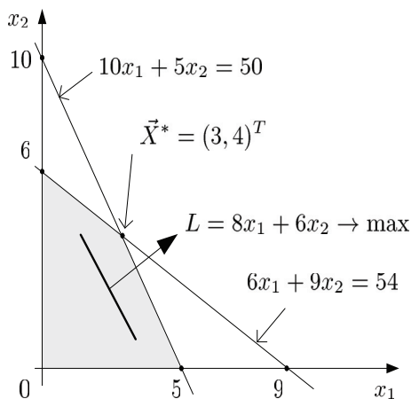
Рис. 4.1. Графическая интерпретация задачи о производственном плане
