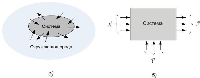
Рис. 1.3. Выделение системы из окружающей среды
