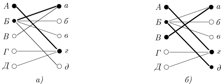
Рис. 7.2. Инверсия чередующейся цепи
