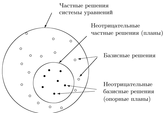
Рис. 4.3. Классификация частных решений системы уравнений
